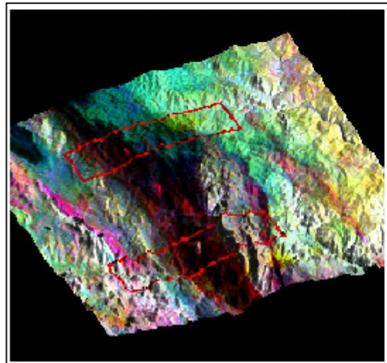
Radiometrics over DEM
